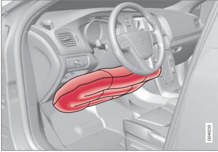
الوسائد الهوائية الخاصة بالركبة في جانب السائق في سيارة ذات عجلة قيادة يسرى.
