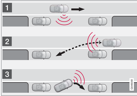
مبدأ وظيفة مرشد مساعد الركن (PAP).
