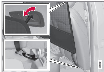
Montage vorn.
