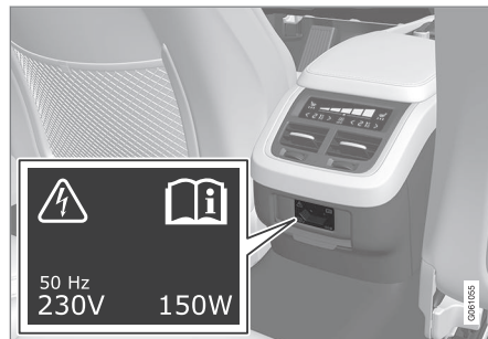
Presseletrica da 230 V nel tunnel, sedile posteriore.
