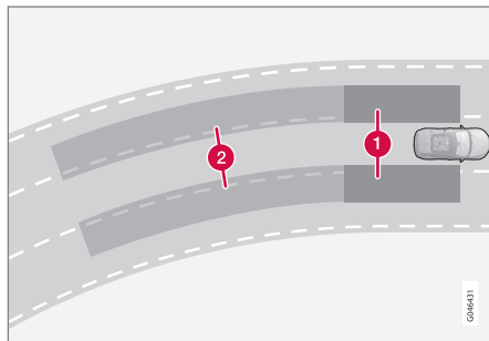
Principi per BLIS; 1. Area nell'angolo morto. 2. Area per veicoli che sorraggiungono rapidamente.
