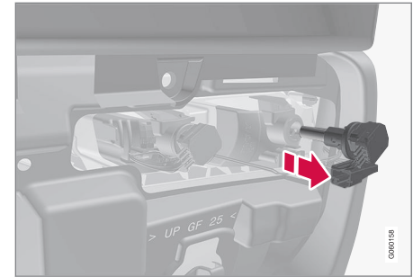
Lamphuis aan de linkerzijde.
