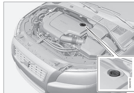
Påfyllningsrör 3 .
