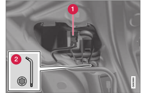
Lamphus på höger sida med täcklock.
