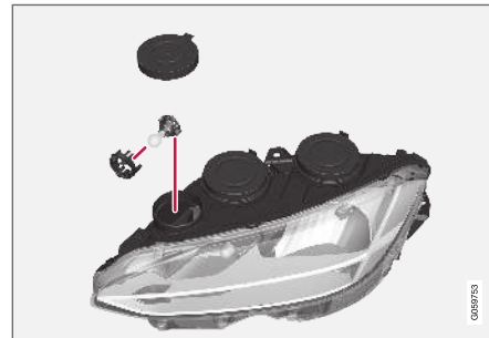
Vänster strålkastare.
