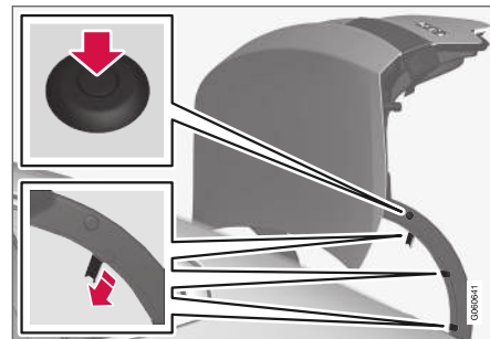
Gångjärnets plasticskydd är monterat med en plastnit och tre snäpplås.
