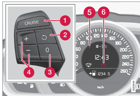
速度リミッター 2 非装備の車両のステアリングリモコンとコンパインド・メーター・パネル
