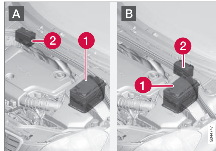
A: soldan direksiyonlu araç. B: Sağdan direksiyonlu araç. (1) Marş aküsü 14 (2) Destek aküsü.
