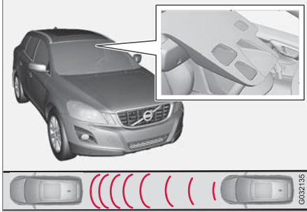
مرسلة مستشعر الليزر ونافذة المستقبل ١٢ .
