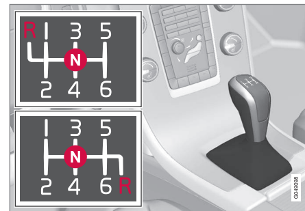
Схема перемикання передач 6-ступінчата КПП.
