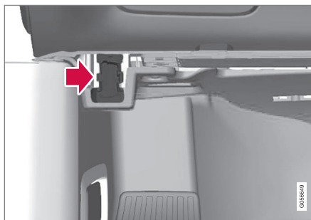
Диагностическое гнездо (гнездо On-board Diagnostic, OBDII) под приборной панелью на сиденье водителя.
