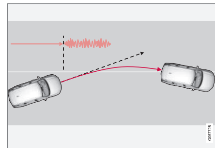
Функция предупреждения о сходе с занимаемой полосы предупреждает водителя вибрацией рулевого колеса.
