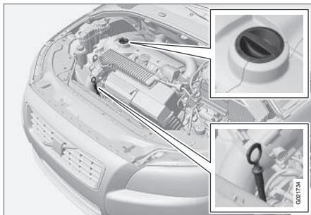
Масляний щуп та маслозаливна горловина.
