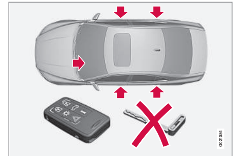
Verriegelungspunkte für Transponderschlüssel ohne Schlüsselblatt und aktivierter Geheimverriegelung.
