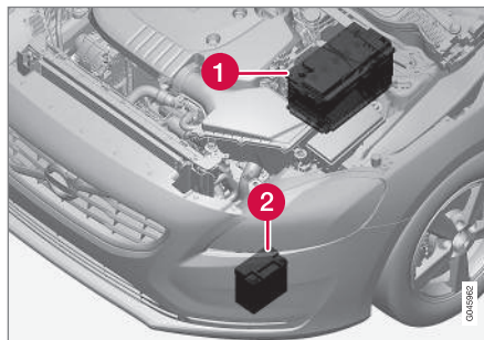
(1) Startaccu 14 (2) Hulpaccu
