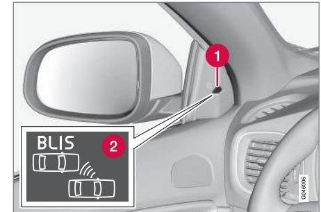
Positie BLIS-lampje 38 .
