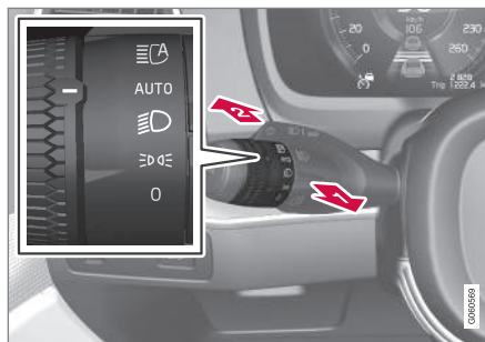
Lever au volant avec molette.
