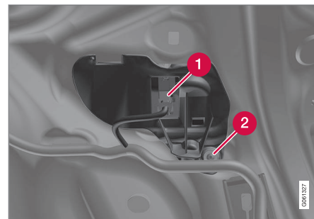
Boîtier de lampe sur le côté droit avec cache.
