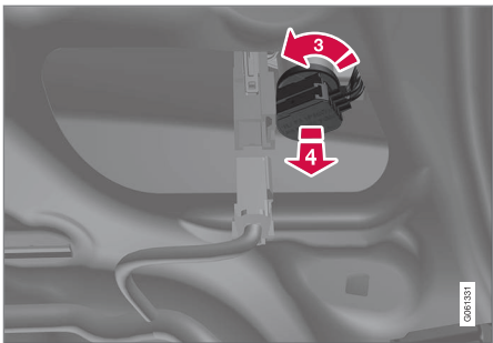
Boîtier de lampe, côté droit.
