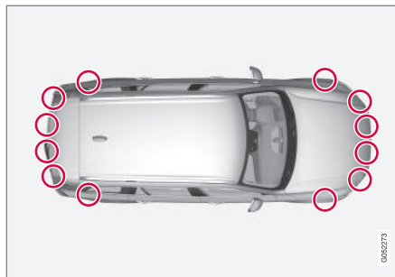
Emplacement des capteurs de PAP 29 .
