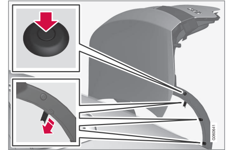
La protection plastique de la charnière est fixée avec un rivet en plastique et trois attaches.
