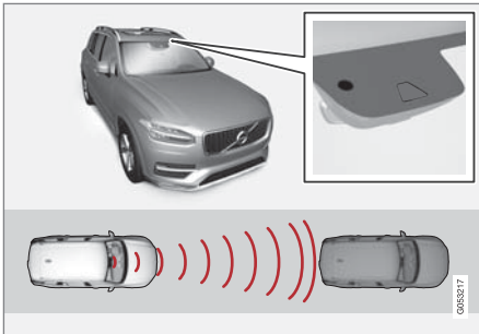
ถัดและชุดเรดาร์จะวัดระยะห่างจากรถคันหน้า 5
