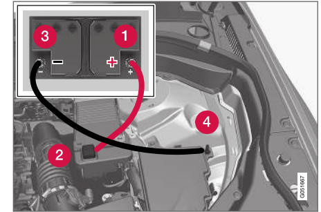
Punkty mocowania przewodów rozruchowych.
