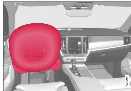
Poduszka powietrzna w kierownicy i kolanowa poduszka powietrzna 1 przy przednim fotelu po stronie kierowcy.
