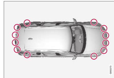
Posizione dei sensori di parcheggio 131 .
