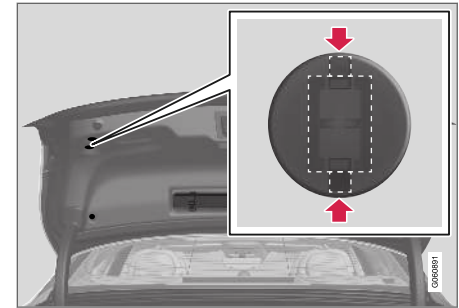
De clips liggen met het rechthoekige deel in de lengterichting van de auto.
