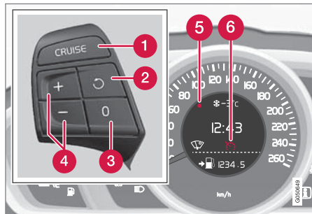
速度リミッター 2 の車両のステアリングリモコンとコンパインド・メーター・パネル
