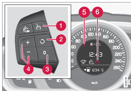
速度リミッター 2 の車両のステアリングリモコンとコンパインド・メーター・パネル
