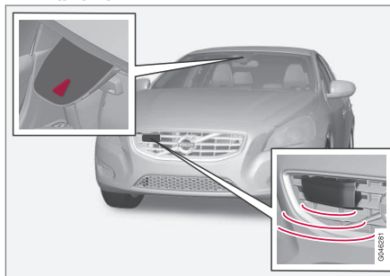
Αισθητήρας κάμερας και αισθητήρας ραντάρ 21 .
