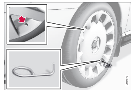
Attrezzo di rimozione dei cappucci in plastica delle colonnette.
