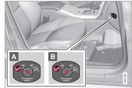
Locatie van de schakelaar voor de airbag.
