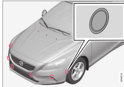
Os sensores PAP estão instalados nos pára-choques 44 - 6 à frente e 4 atrás.
