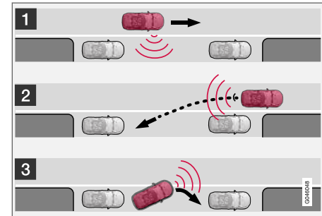
Princípio de funcionamento do PAP.
