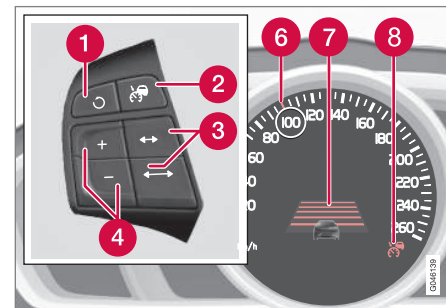
Адаптивный круиз-контроль без ограничителя скорости 9 .
