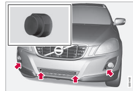
Расположение передних датчиков.
