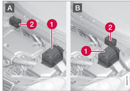
A: soldan direksiyonlu araç. B: Sağdan direksiyonlu araç. (1) Marş aküsü 17 (2) Destek aküsü.
