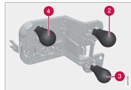
Porte-lampe de feu rouge arrière
