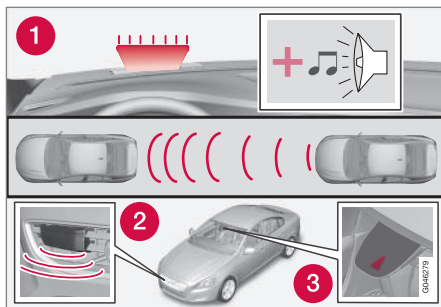
Elementy układu 22 .
