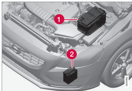
(1) Akumulator rozruchowy 14 (2) Akumulator pomocniczy
