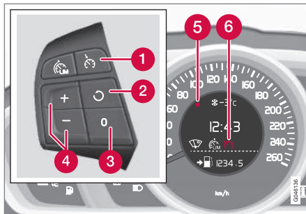
Teclado do volante e mostrador no automóvel com Limitador de velocidade 9 .
