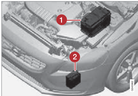
(1) แบตเตอรี่สตาร์ท 17 (2) แบตเตอรี่เสริม
