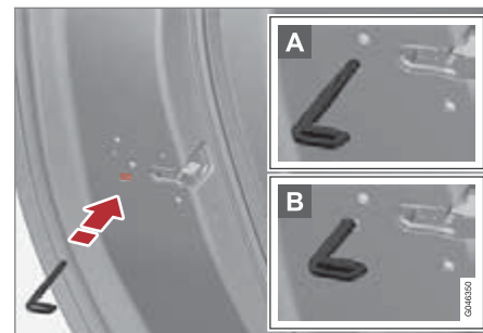
การล็อคประตูด้วยมือ อย่าสับสนกับล็อคนิรภัยสำหรับเด็ก (น. 219)
