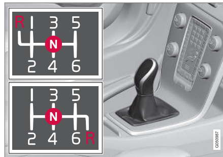
Układ biegów.
