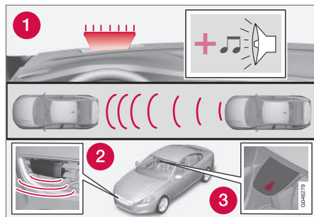
Elementy układu 22 .
