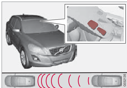
雷射感知器發射器與接受器的視窗 18 。
