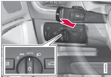
頭燈控制之調整桿及旋鈕在 AUTO 位置。
