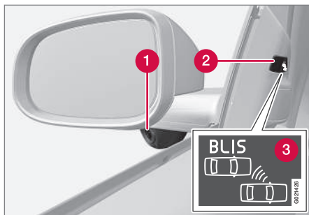
Buitenspiegel met BLIS 34 .
