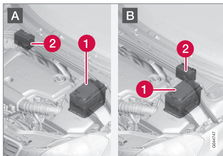
A: Automóvil con volante a la izquierda. B: Automóvil con volante a la derecha. (1). Batería de arranque 17 (2). Batería de apoyo.
