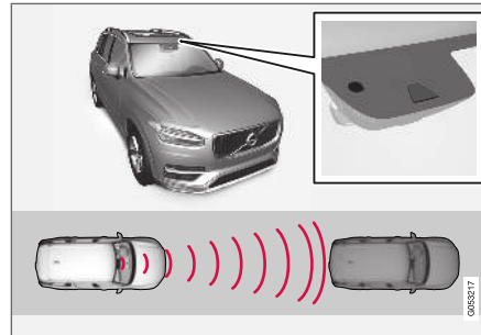
Umiejscowienie modułu radarowego 80 .
