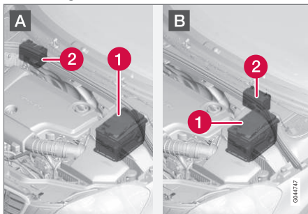
A: Modelos com volante à esquerda. B: Modelos com volante à direita. (1) Bateria de arranque 19 (2) Bateria de apoio.
