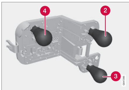
Suporte da lâmpada da luz traseira
