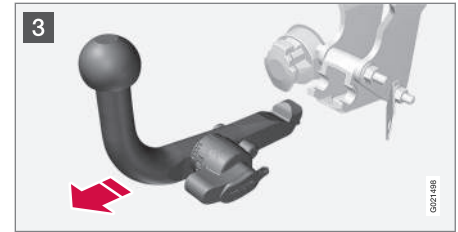
3 Gire hacia abajo la rueda de cierre por completo hasta el tope y retenga al mismo tiempo el enganche para remolque, que debe sacarse hacia atrás y hacia arriba.
