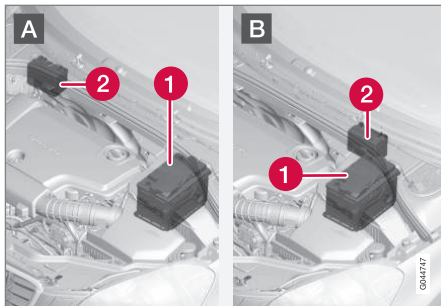
A: Vozidlo s levostranným řízením. B: Vozidlo s pravostranným řízením. (1). Startovací baterie 12 (2). Pomocná akumulátor.
