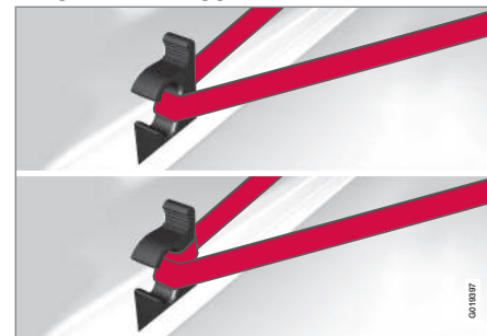
Fissaggio del carico con ganci fermacarico mobili .
