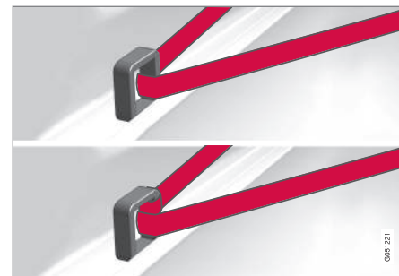
Fissaggio del carico con occhielli fermacarico fissi .
