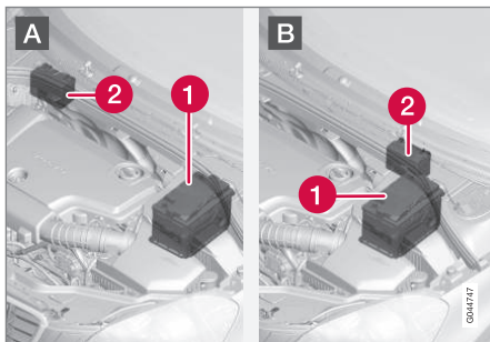
A: Auto met stuur links. B: Auto met stuur rechts. (1) Startaccu 19 . (2) Hulpaccu.
