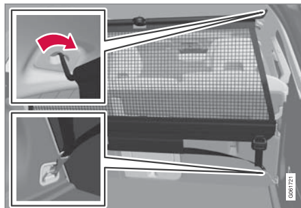
뒤쪽 고정.
