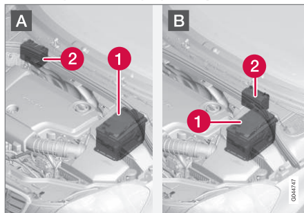
А: Лівостороннє кермо. В: Правостороннє кермо. (1) Акумулятор стартера 17 (2) Допоміжний акумулятор.
