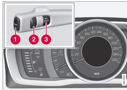
Дисплей (аналогова комбінована панель приладів) і органи керування навігацією в меню.
