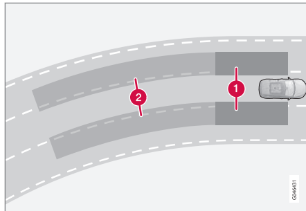
Принцип роботи BLIS: 1. Мертва зона. 2. Зона розпізнавання автомобілів, що швидко наближаються.
