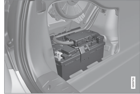
Marş motoru aküsü kargo alanında bulunur.
