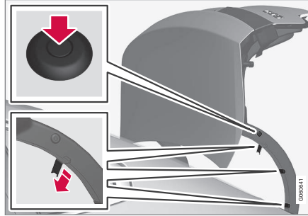
Menteşenin plastik korumasına plastik bir perçin ve üç mandal takılır.
