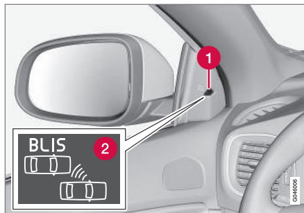
Positie BLIS-lampje 23 .
