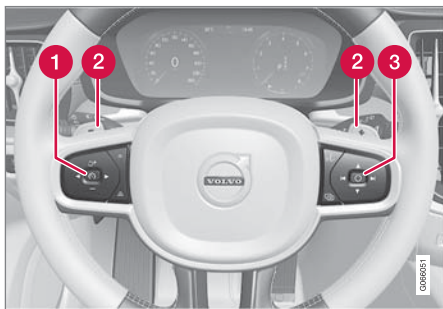
方向盤上的鍵盤與撥片*。
