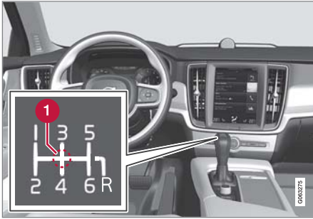
ภาพรวมของคันเกียร์และตำแหน่งการเปลี่ยนเกียร์
