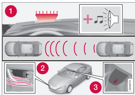
Vista general de la función 13 .
