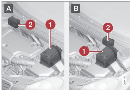
A：左駕車。B：右駕車。(1) 起動電瓶 16 (2) 支援電瓶。
