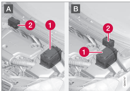
A: Bil med vensterratt. B: Bil med høyerratt. (1.) Startbatteri 16 (2.) Hjelpebatteri.
